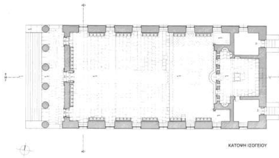
Κάτοψη
