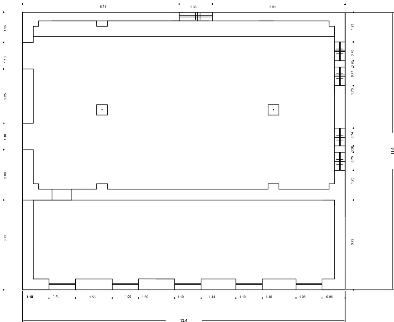
Κάτοψη Ισογείου
