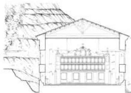
ΤΟΜΗ ΑΑ
